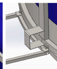
Установка лестницы с трапом для обрешеток TRF
