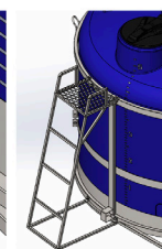
Установка лестницы с трапом для обрешеток TRF
