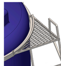
Установка лестницы торцевой с трапом для обрешеток TRF
